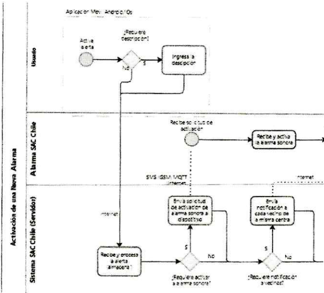
Modelamiento de proceso principal de Sistema SAC Chile
