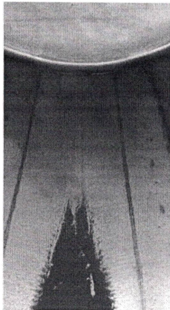
Presencia de corrosión al interior de TK de RTHX-98, se debe eliminar.
