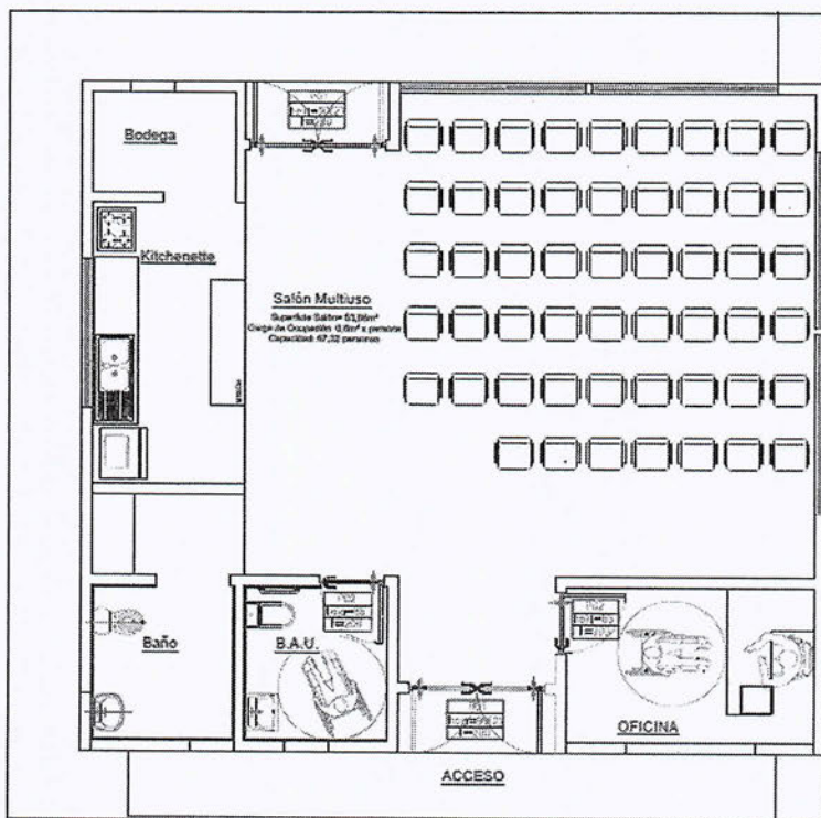
Planta de Arquitectura
